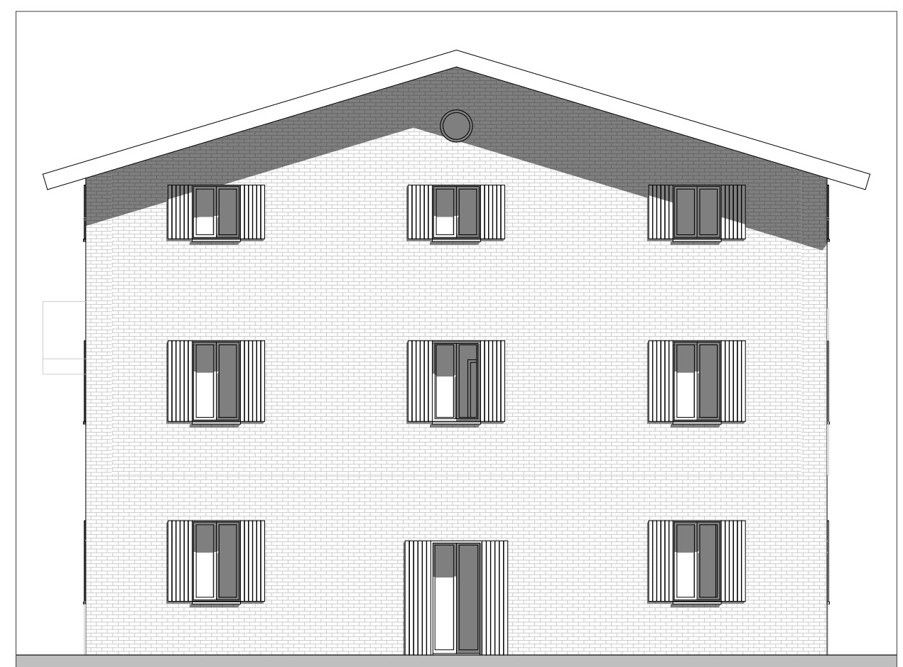
OVEST 1 1:100
