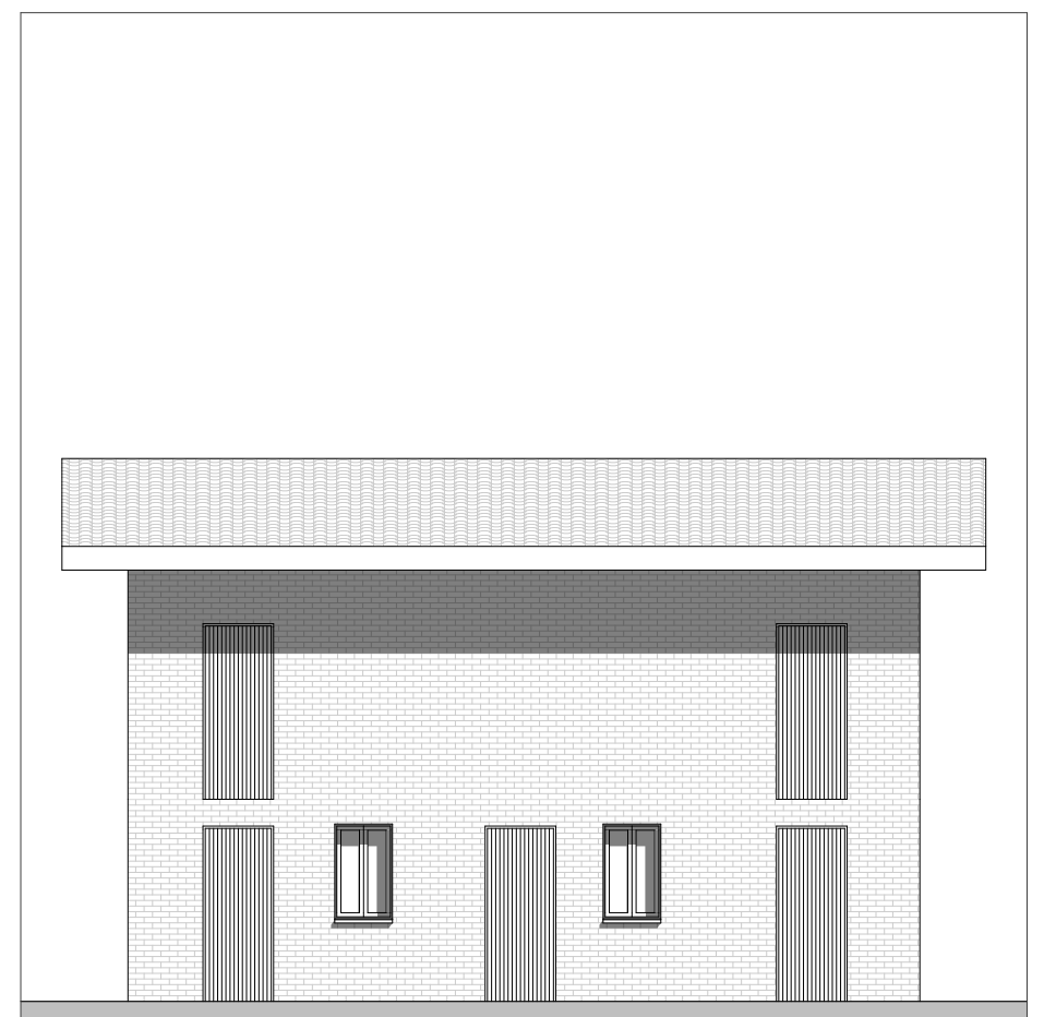
OVEST 2 1:100
