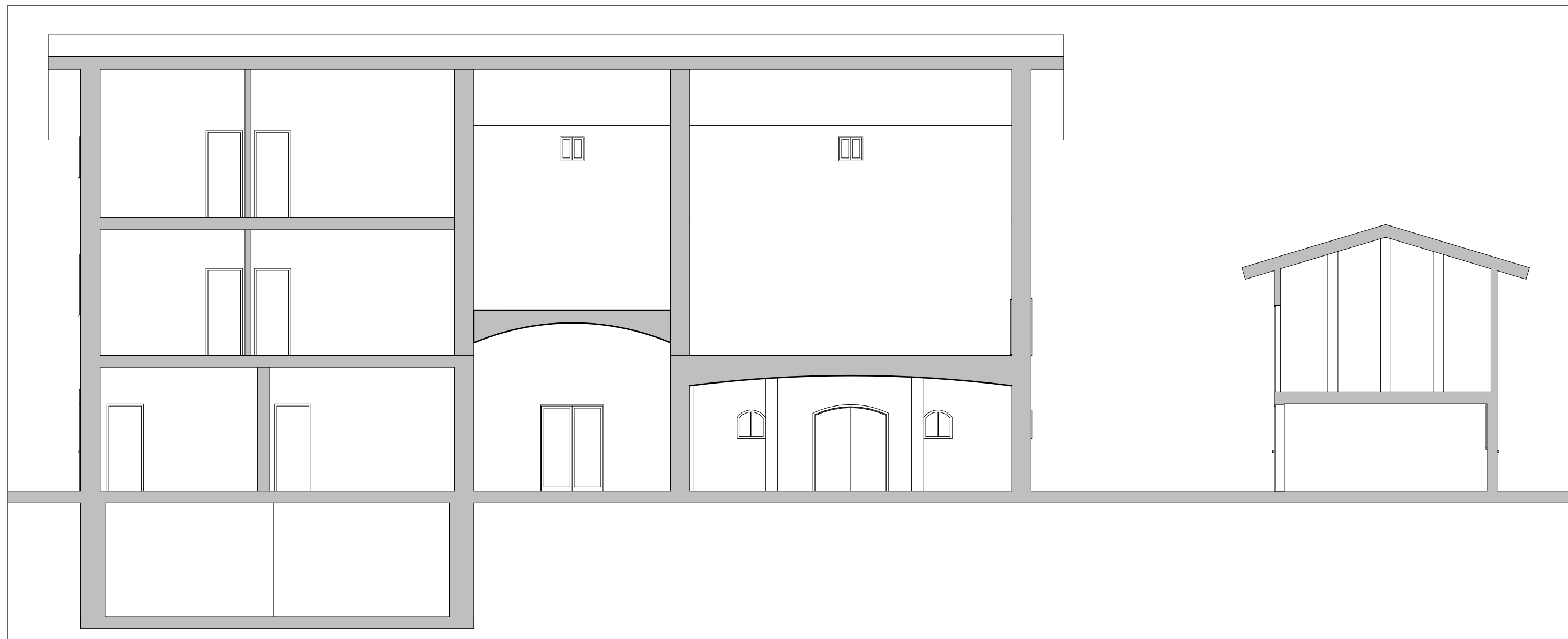
A Sezione longitudinale 1:100
